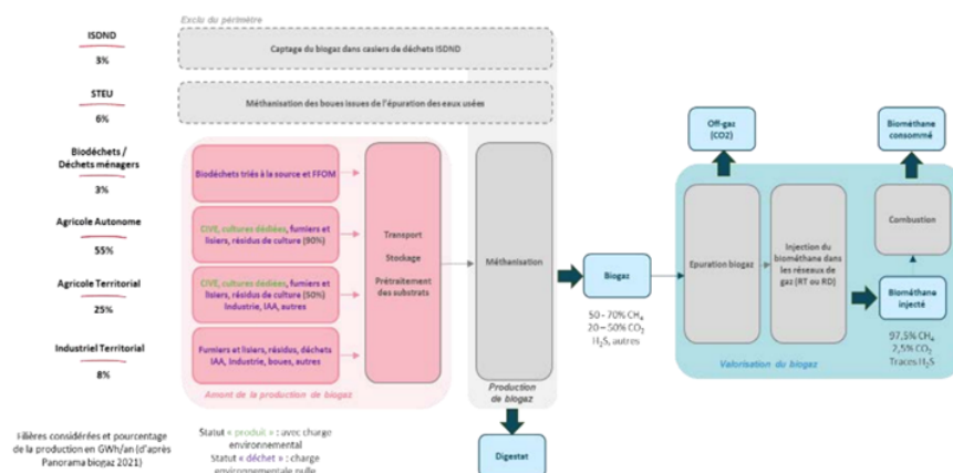
Figure 1 - Schéma macro simplifié des différentes filières de production de biométhane en France.
